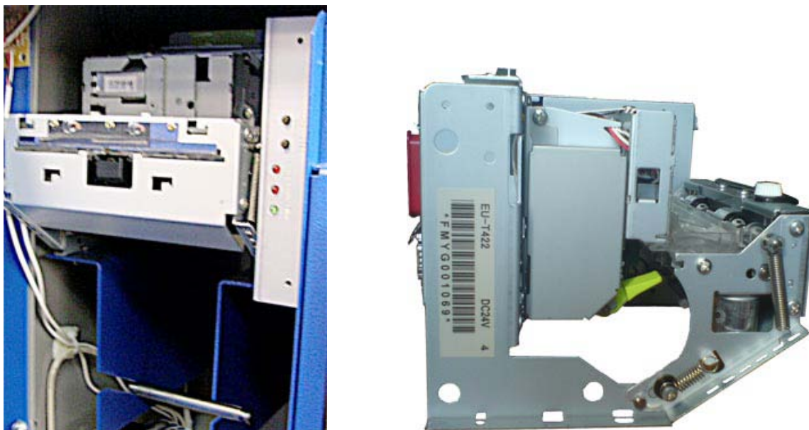
Рис. 25. Замена термобумаги
