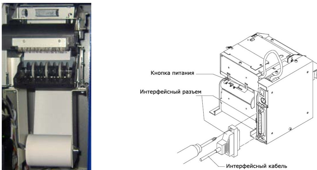
Рис. 22. Внешний вид принтера Citizen PPU-700
