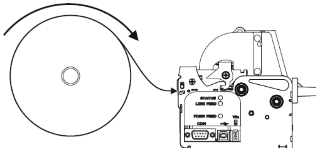
Рис. 27. Замена термобумаги
