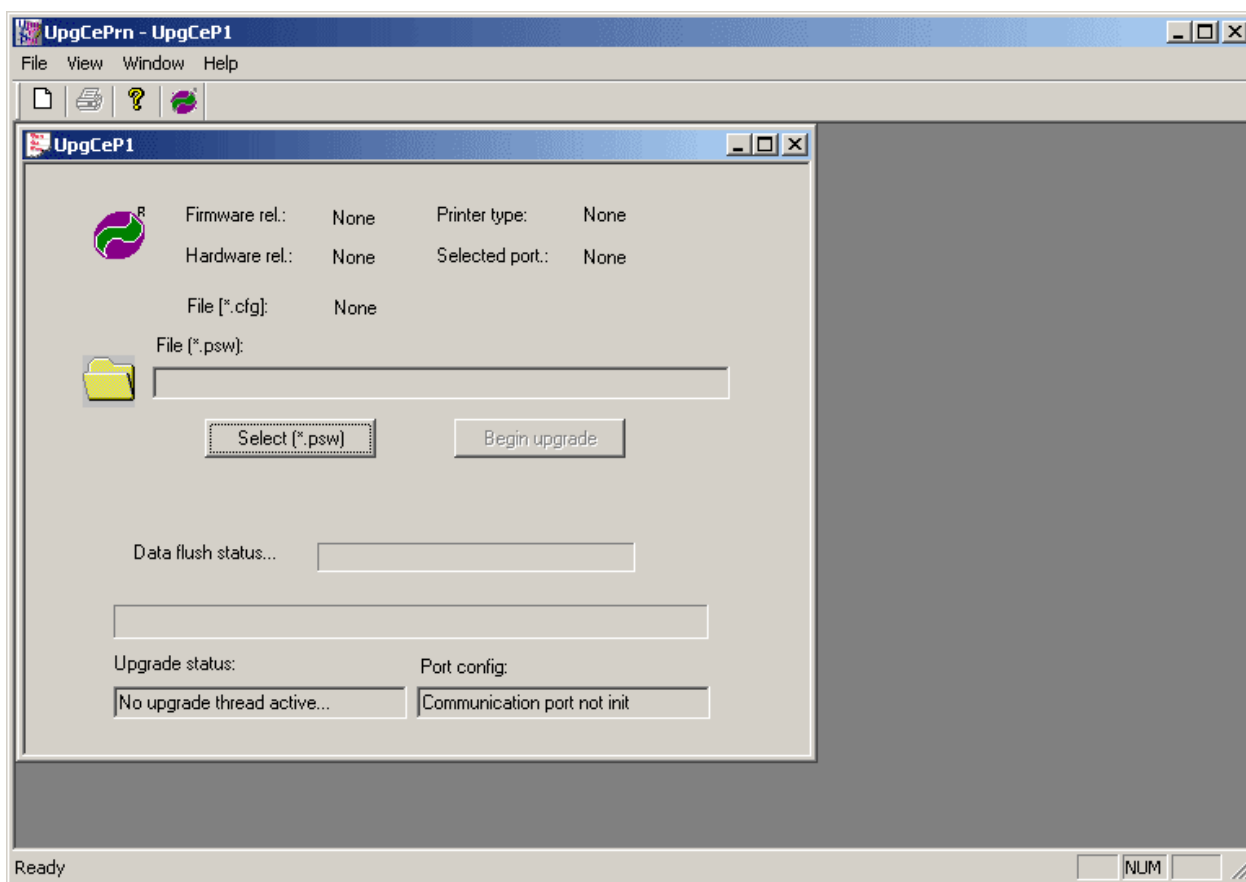
Рис. 28. Программа «UpgCePrn»
