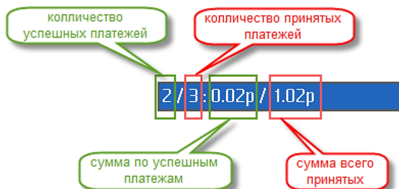
Рис. 14. Заголовок окна «Статусы»
