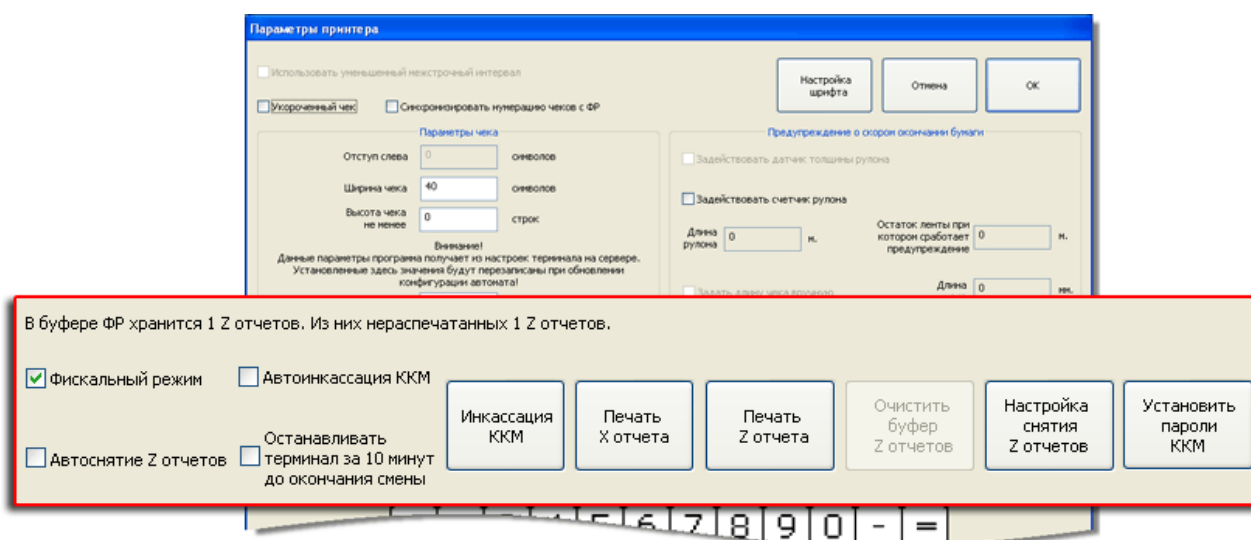
Рис. 8. Фискальный режим
