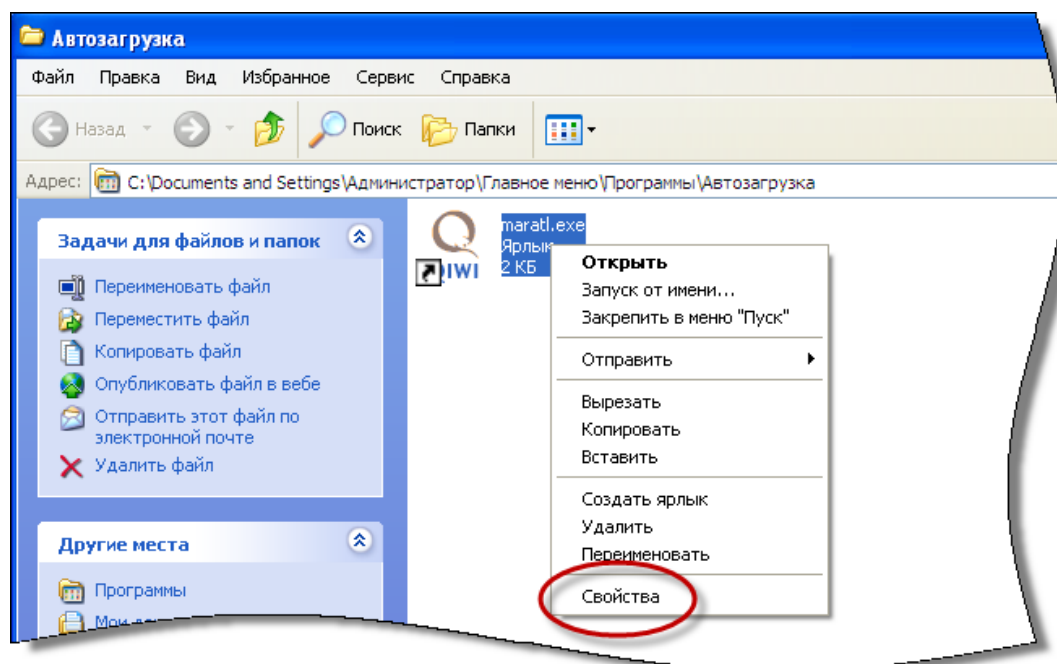
Рис. 17. Контекстное меню
