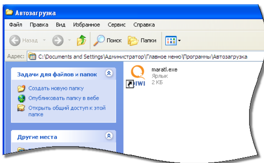
Рис. 16. Папка «Автозагрузка»
