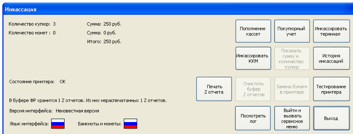
Рис. 9. Диалог «Инкассация»
